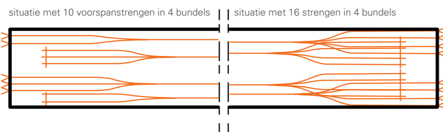
Figuur 1 Schematische weergave verloop voorspanstrengen
